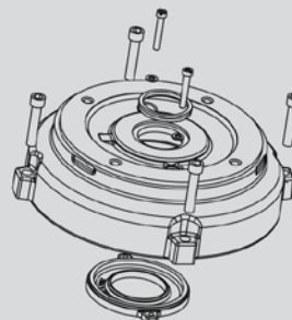
C Flange Kit
